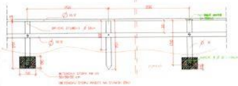
IZGLED OGRADE
